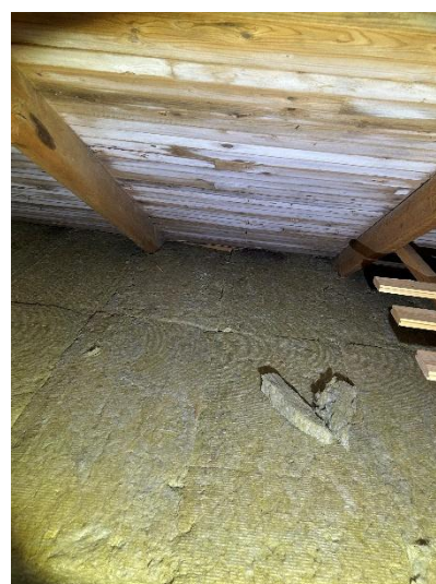
Vid stickprov i underlagstaket noterades 10,3%, 8,0% och 8,9%. Missfärgningar, microbiellpåväxt och fuktgenomslag.
